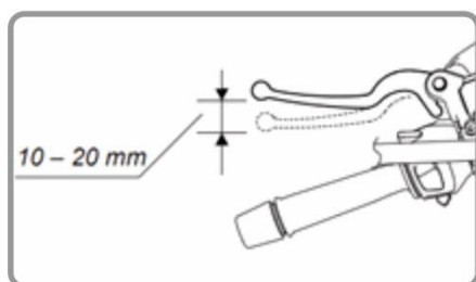
Manete de embraiagem
