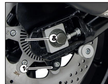
1. Sensor da roda traseira 2. Rotor do sensor traseiro
