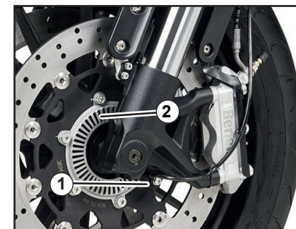
1. Sensor da roda dianteira 2. Rotor do sensor dianteiro
