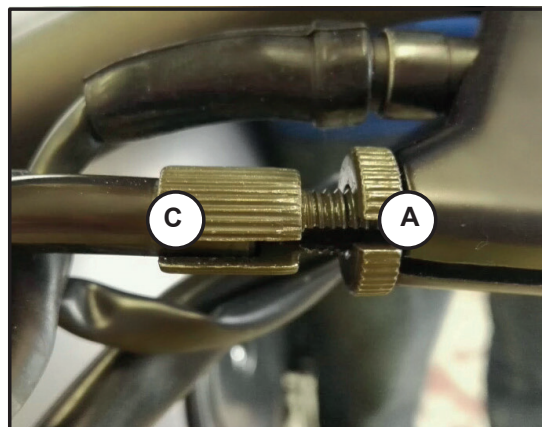
A. Contra porca de afinação C. Parafuso de afinação
